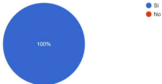
Ilustración 16- Cuestionario pregunta 2
