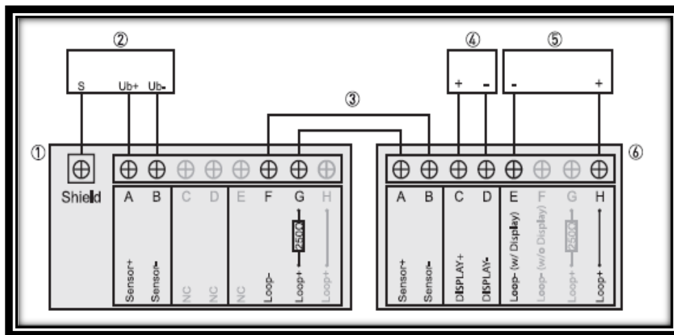
Ilustración 16. Conexión con Sensor y Sistema de Control
