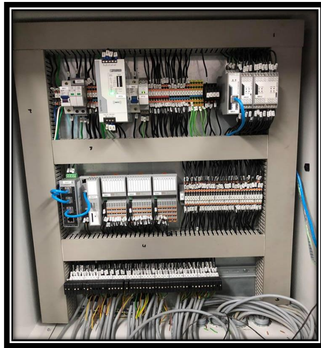
Ilustración 33. Panel de control Planta de Tratamiento, ASP
