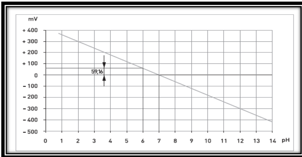
Ilustración 6. Pendiente óptima a 25 ° C / 77 ° F
