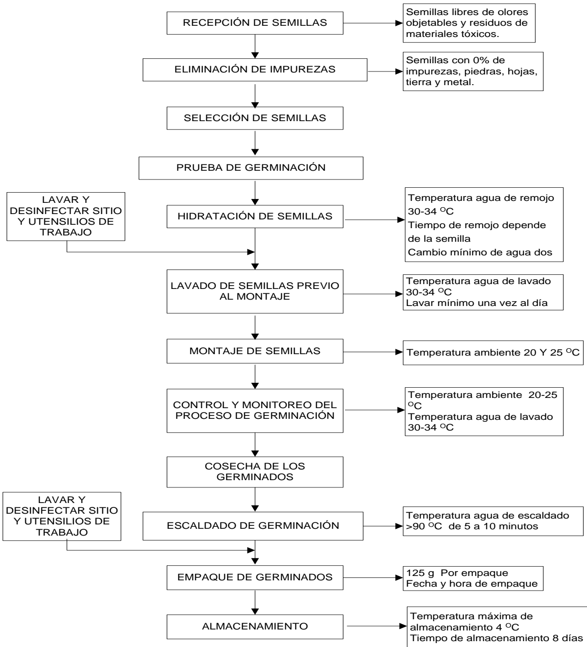
Figura 3. Diagrama de flujo del proceso de obtención de semillas germinadas.
