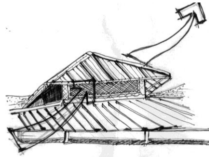
Figura 20. Chimenea de ventilación
