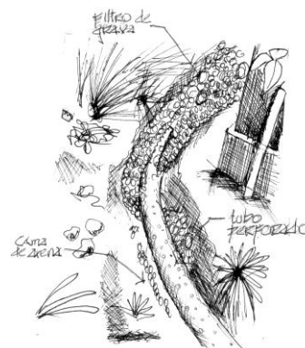
Figura 138. Drenaje Francés
