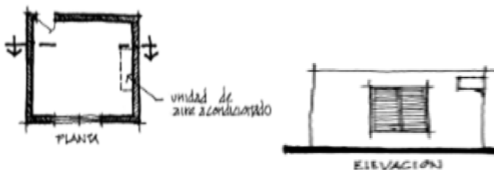
Figura 149 y150. Instalación aire acondicionado en planta y corte.
