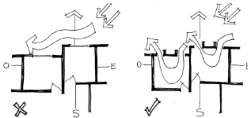
Figura 160. Ventilación cruzada en una sola pared
