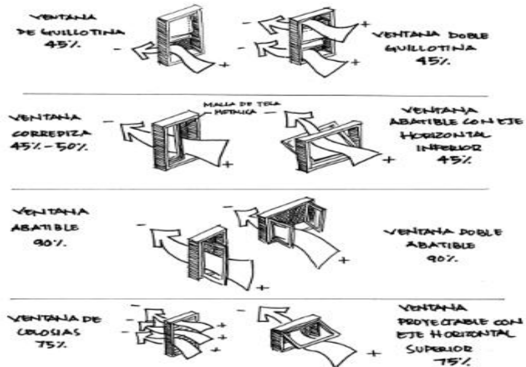
Figuras 77. Efectividad ventilación natural /modelos de ventana
