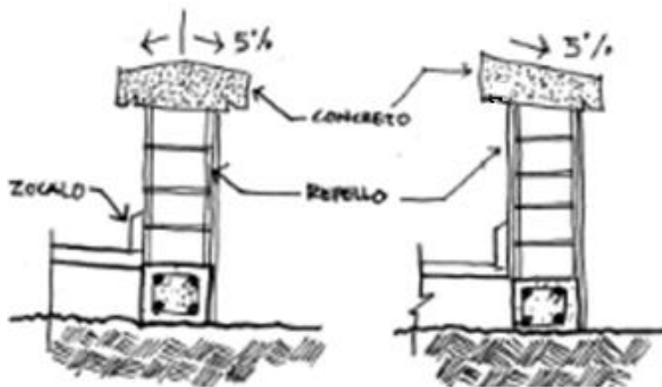
Figura 115. Corta lágrimas en muros
