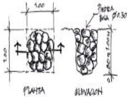
Figura 127. Detalle sumidero
