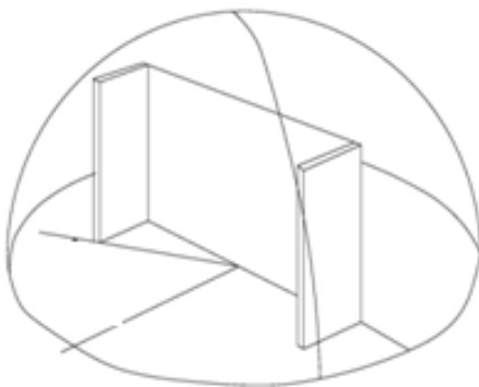
Figura 99. Quebra sol vertical
