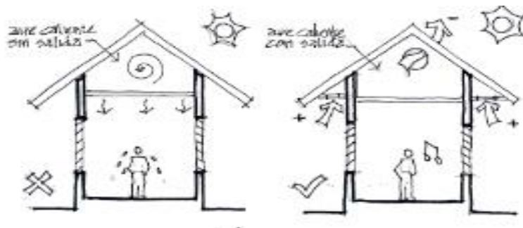
Figura 155. Evacuación de aire caliente entre cielo falso y techo
