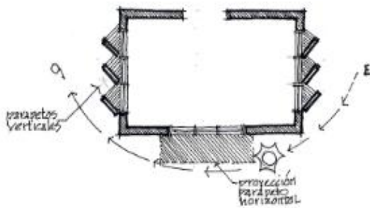
Figura 111. Parapetos inclinados
