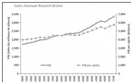
Figura 1 América Latina, 1990-2012: Producto interno bruto (PIB) total y PIB per cápita (a precios de 2005)
