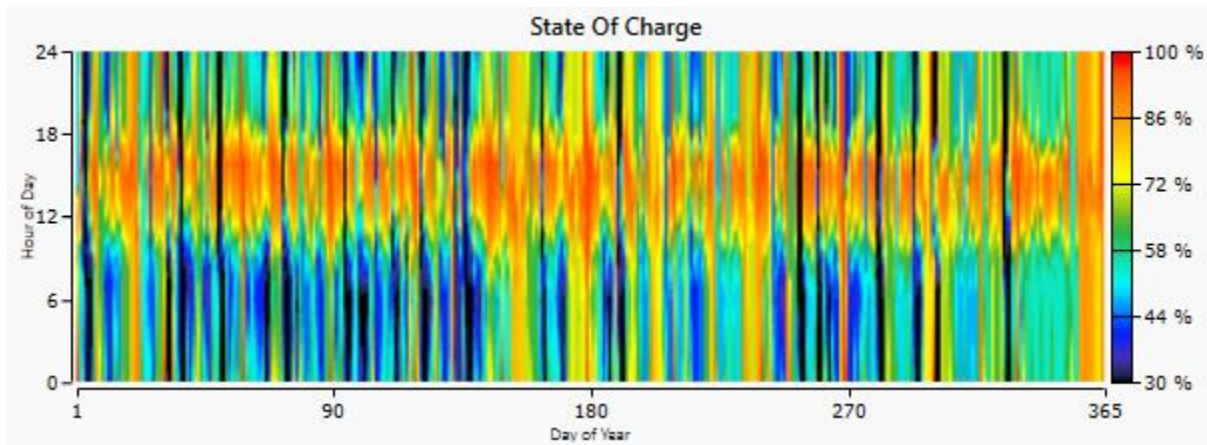
Ilustración 42. Estados de carga del sistema de almacenamiento del escenario 3.
