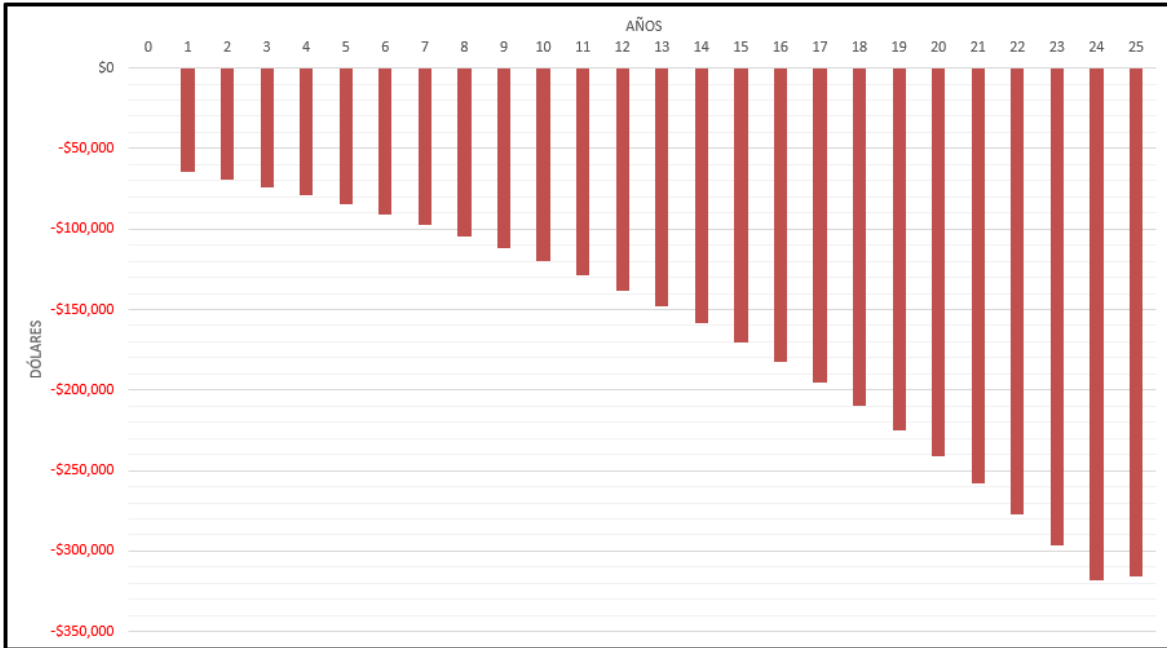
Ilustración 33. Proyección de costos nominales anuales del escenario base.
