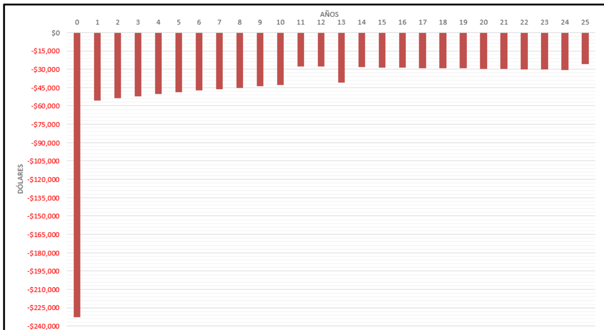
Ilustración 36. Costos anuales descontados del escenario 1.
