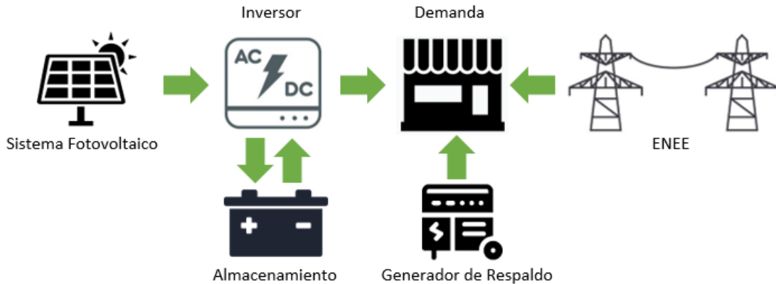
Ilustración 14. Modelo energético del escenario 2.
