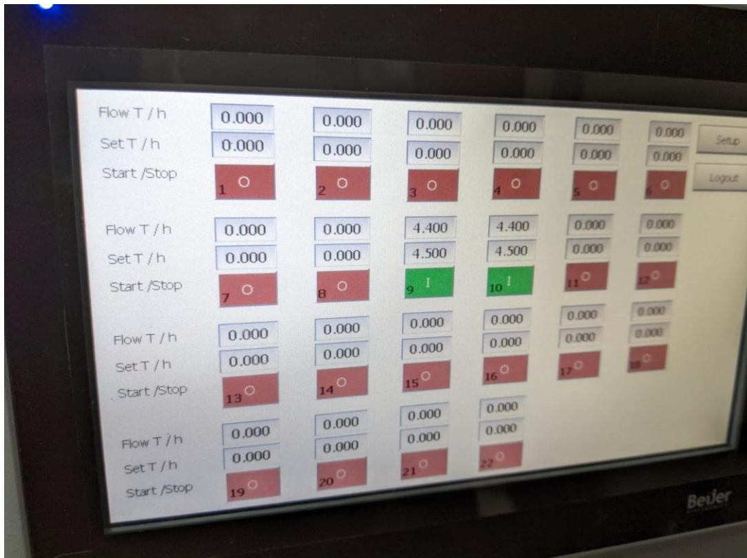
Ilustración 14 HMI en panel de control
