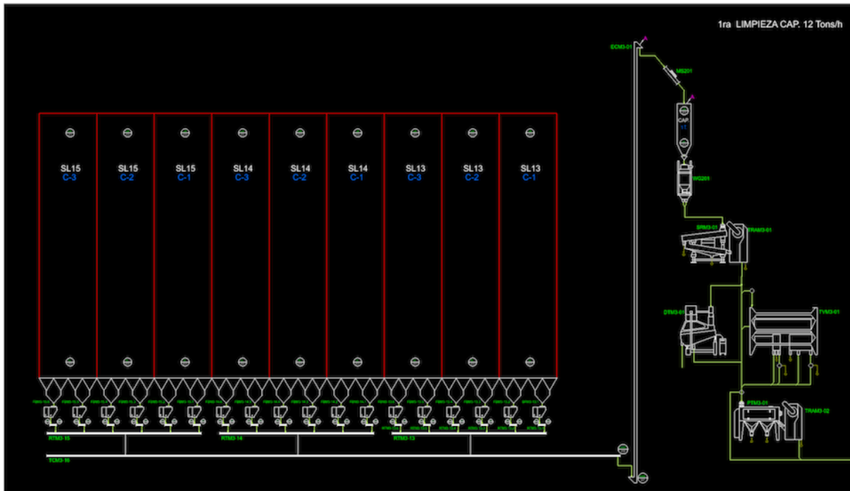
Ilustración 4 Plano de ponderables TFBI bajo silos 13, 14 y 15
