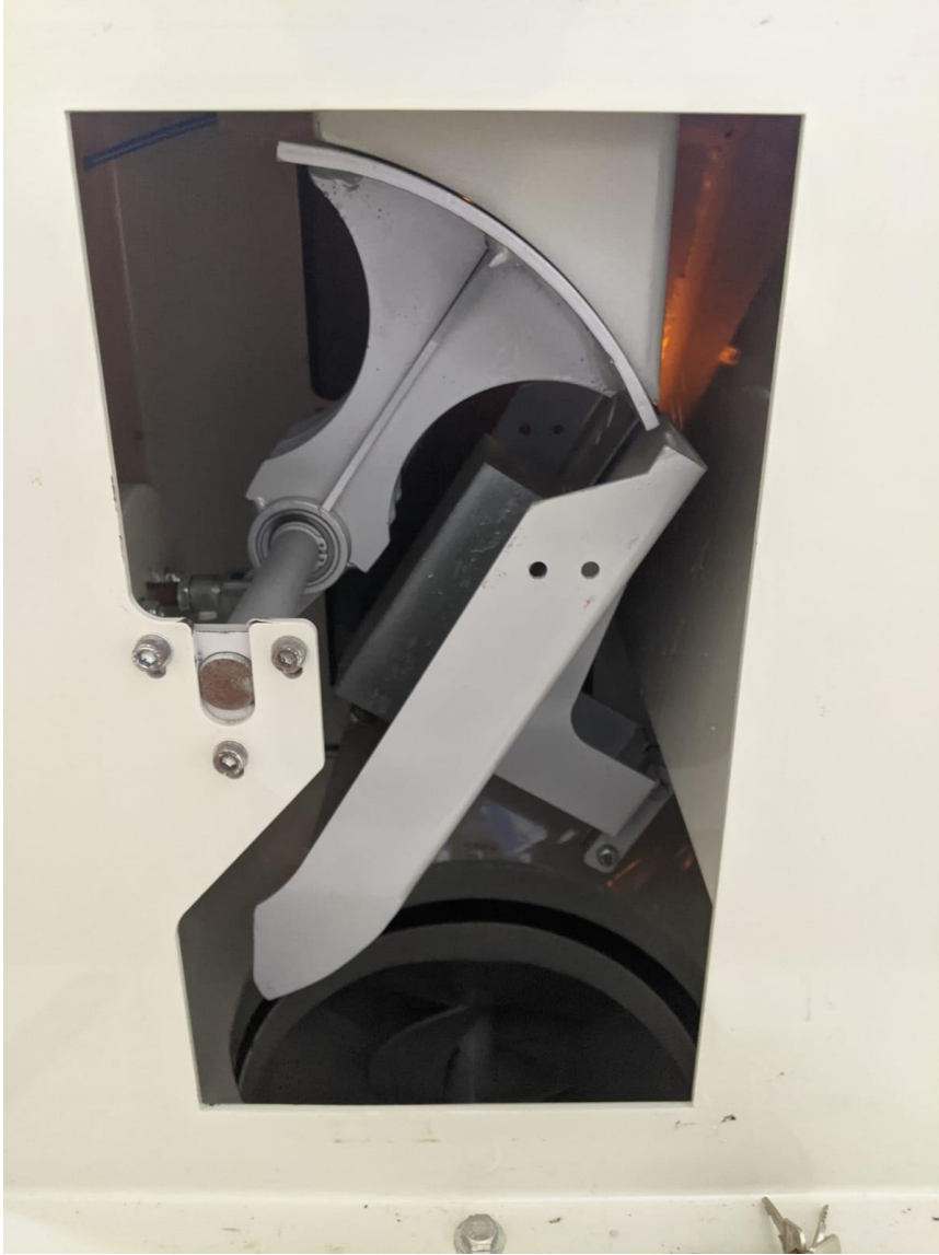
Ilustración 11 Masa de 3kg dentro del Flow Balancer para calibración
