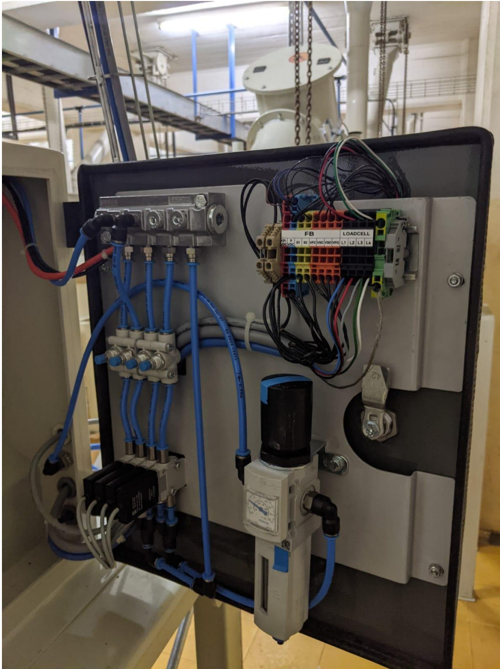
Ilustración 16 Panel de control de valvulas neumáticas de FB
