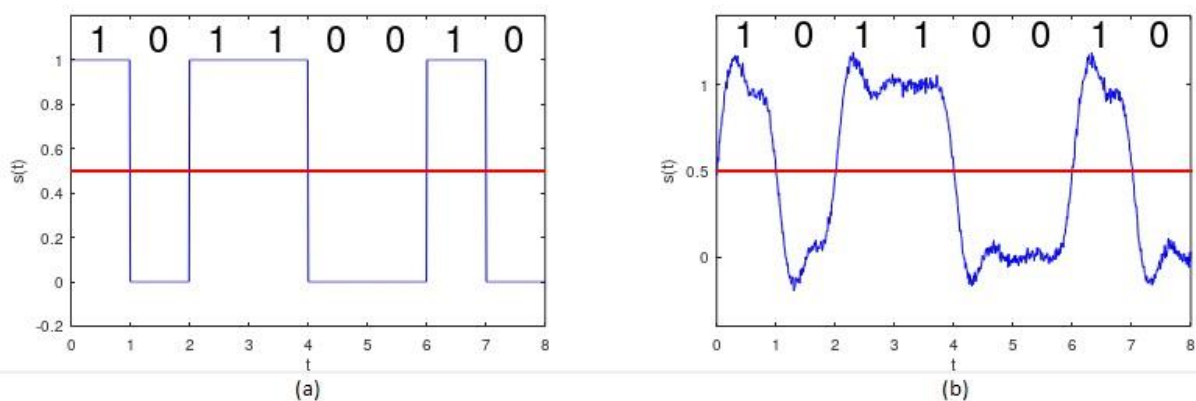
Ilustración 1 Señal digital (a) y Señal analógica (b)
