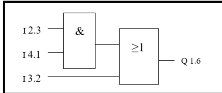
Ilustración 3 Programación por medio de diagrama de funciones
