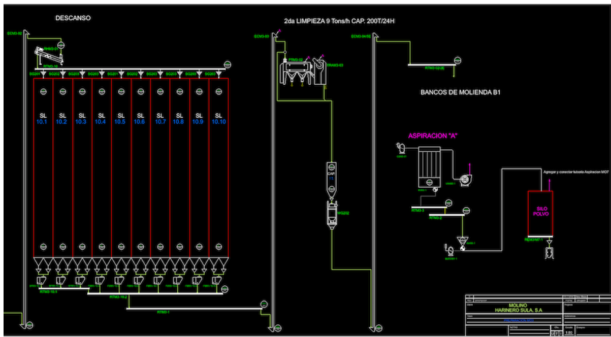
Ilustración 5 Plano de ponderables bajo silo 10 y TOCA sobre silo 10
