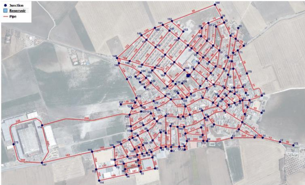
Ilustración 1-Tipología de la red de abastecimiento de agua de los Molares.
