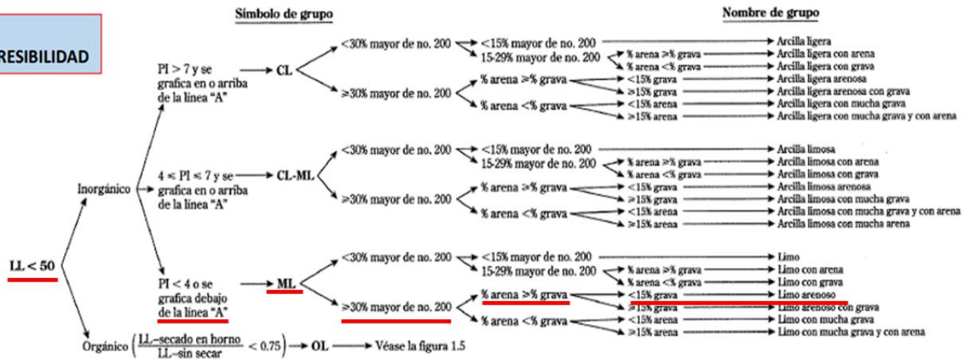
Ilustración 23- Diagrama de clasificación SUCS
