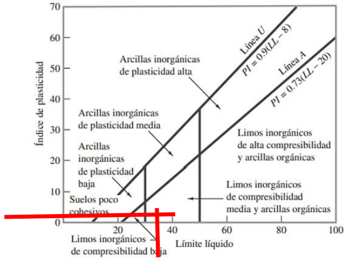
Ilustración 22- Carta de Casagrande
