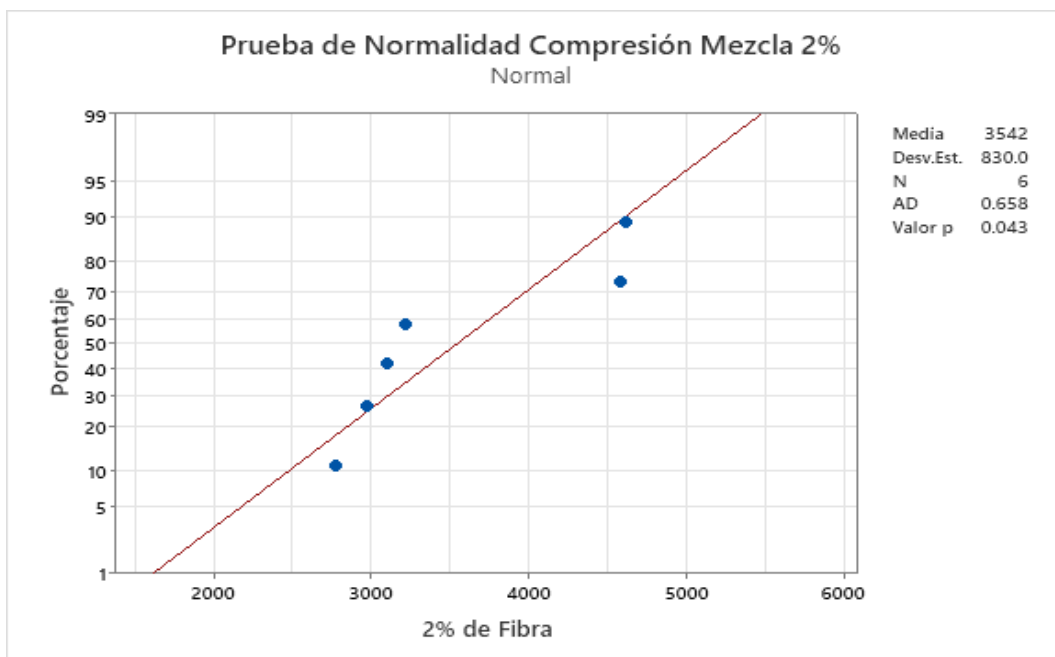
Ilustración 43. Prueba de normalidad de mezcla de concreto con 2% de fibra
