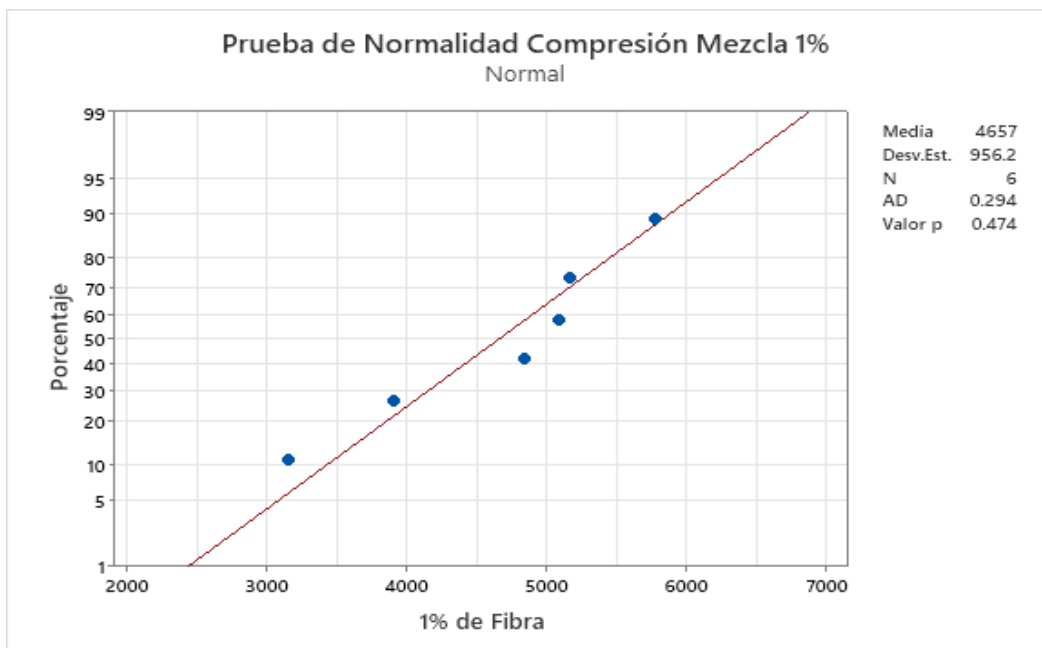
Ilustración 41. Prueba de normalidad a la compresión de mezcla de concreto con 1% de fibra.
