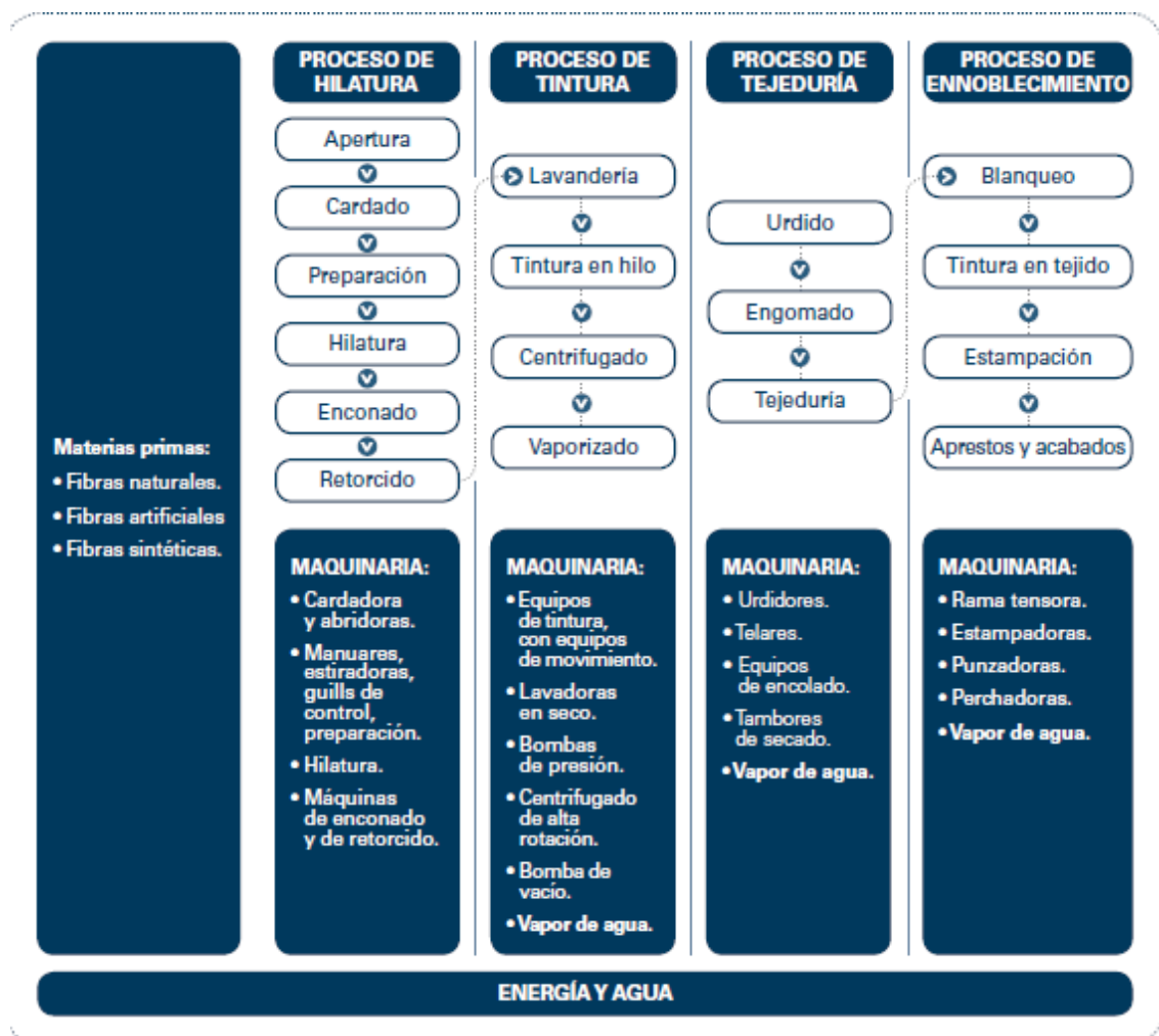
Ilustración 6. Proceso de Producción de la Industria Textil
