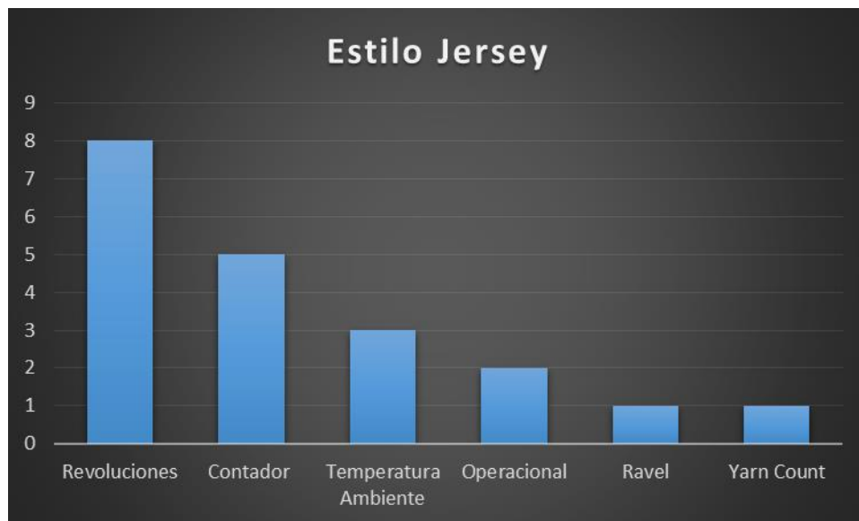
Ilustración 16. Causas de Fallo en las Máquinas
