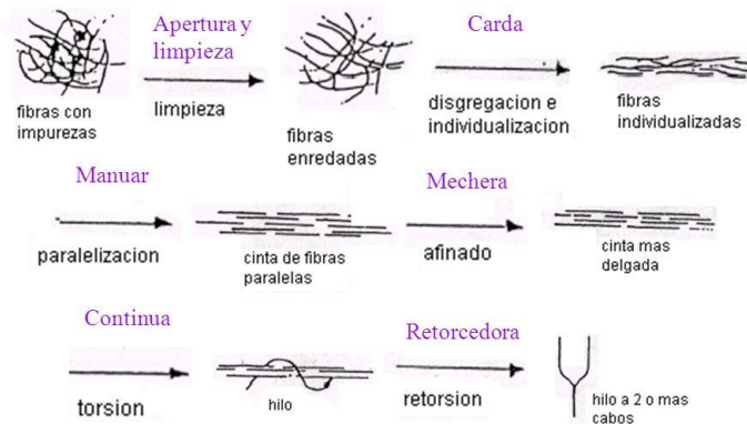
Ilustración 4. Proceso de Hilatura de la Fibra al Hilo
