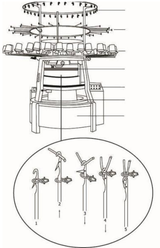
Ilustración 5. Proceso de Tejeduría Mediante Máquinas Circulares
