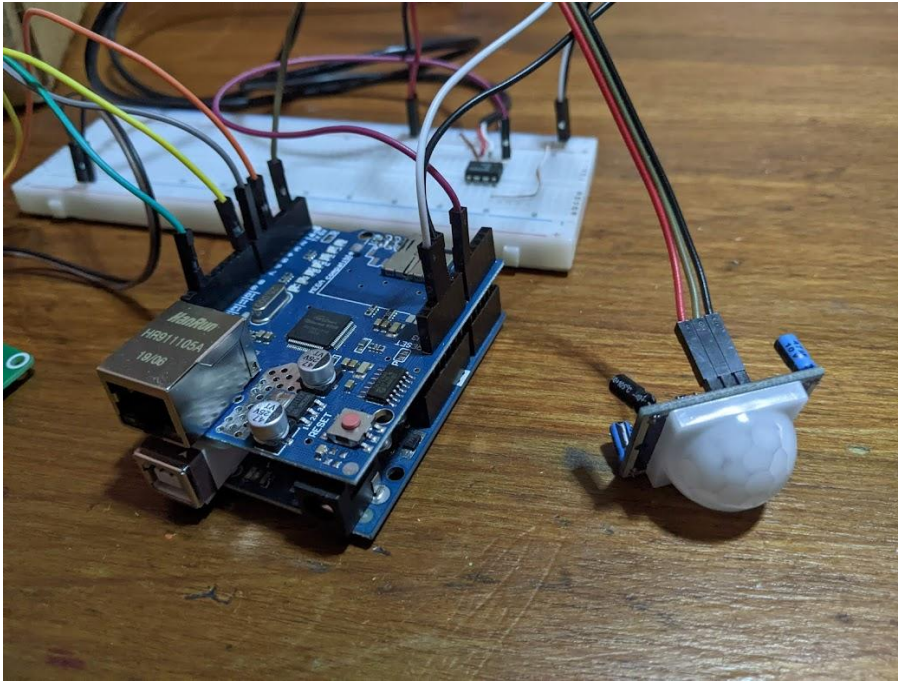
Arduino y Sensor PIR HC-SR501
