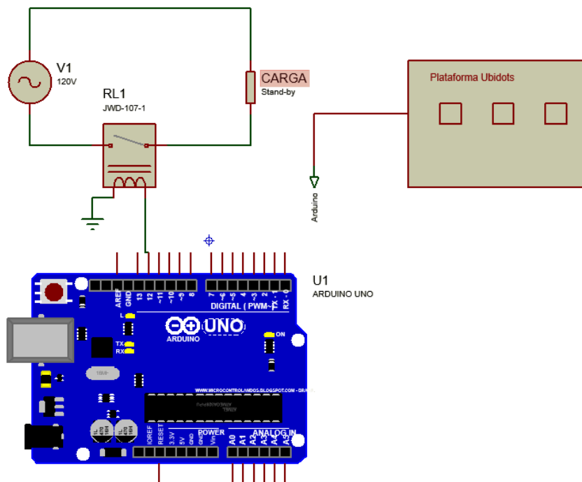
Figura 6.6 Conexión del circuito controlador de dispositivos en Stand-by
