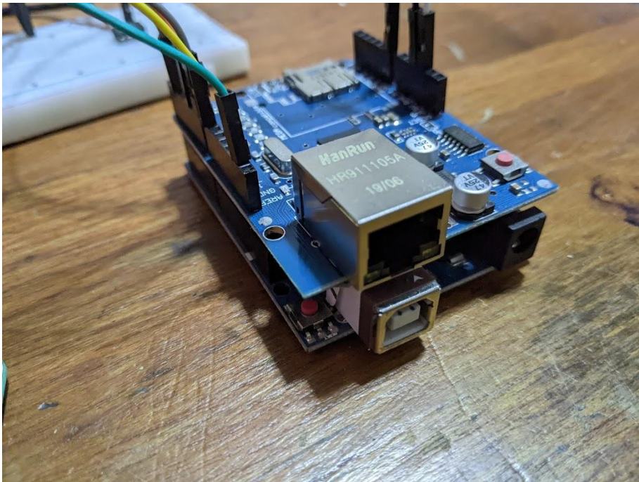
Arduino UNO y módulo Ethernet W5100
