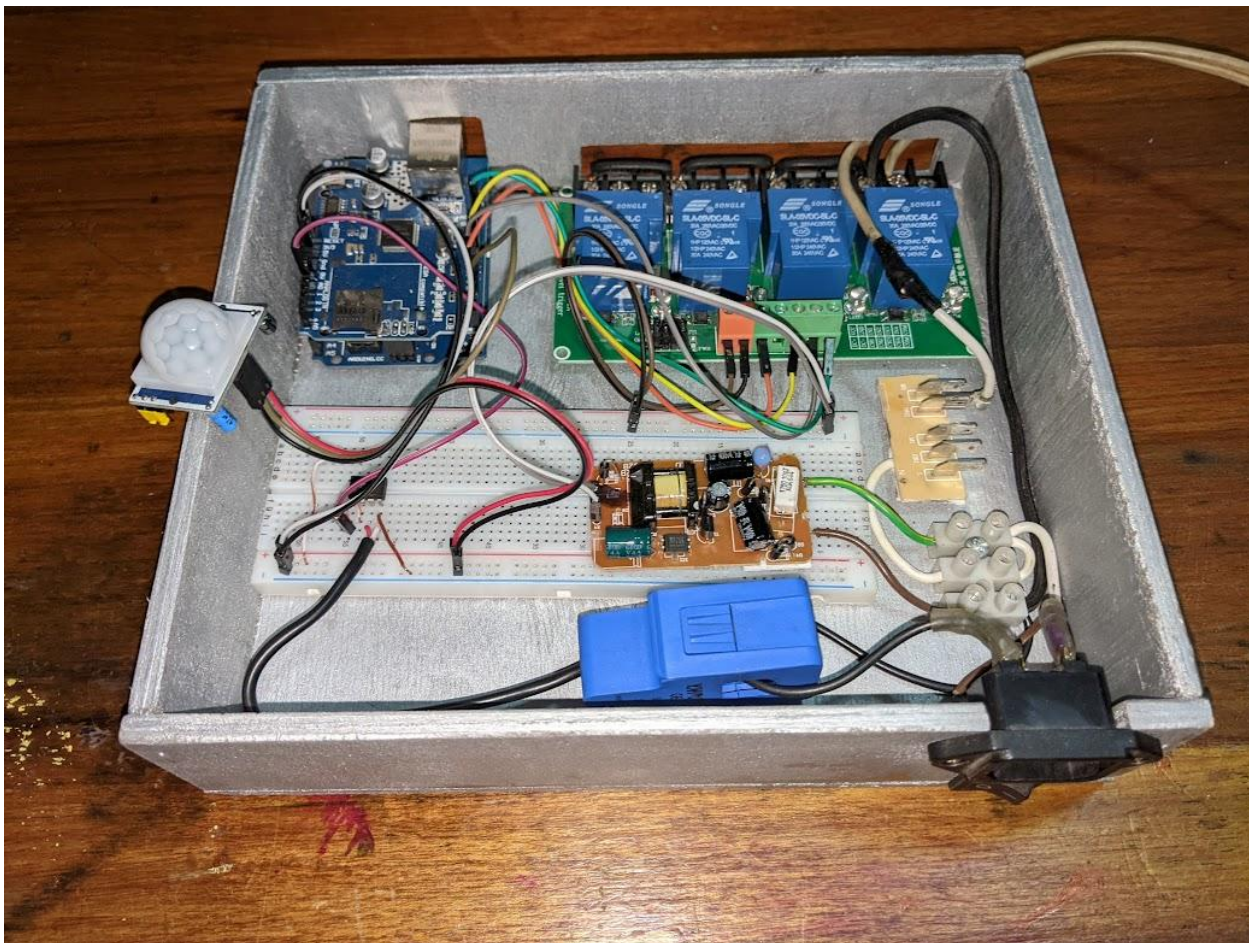
Figura 8.27 Montaje del prototipo
