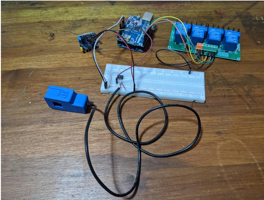
Montaje de prototipo
