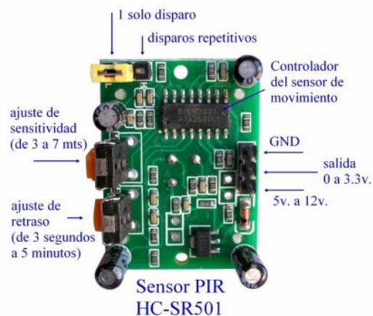
Figura 8.22 Conexiones del módulo sensor PIR HC-SR501
