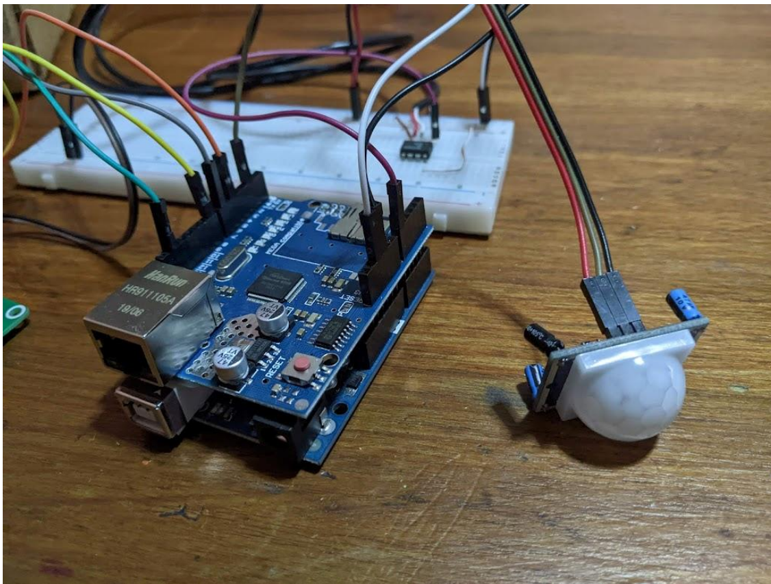
Figura 8.24 Montaje del controlador de iluminación en el prototipo
