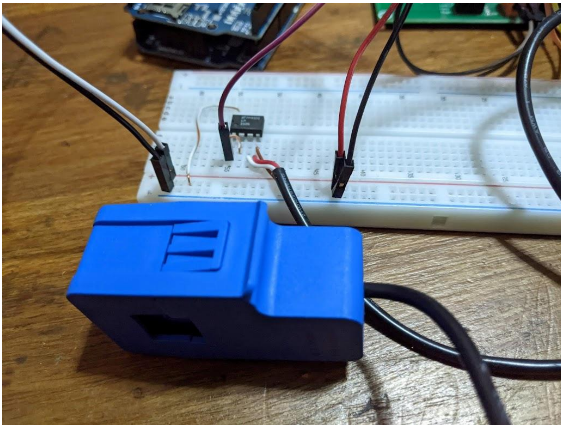
Figura 8.20 Montaje del medidor de consumo en el prototipo
