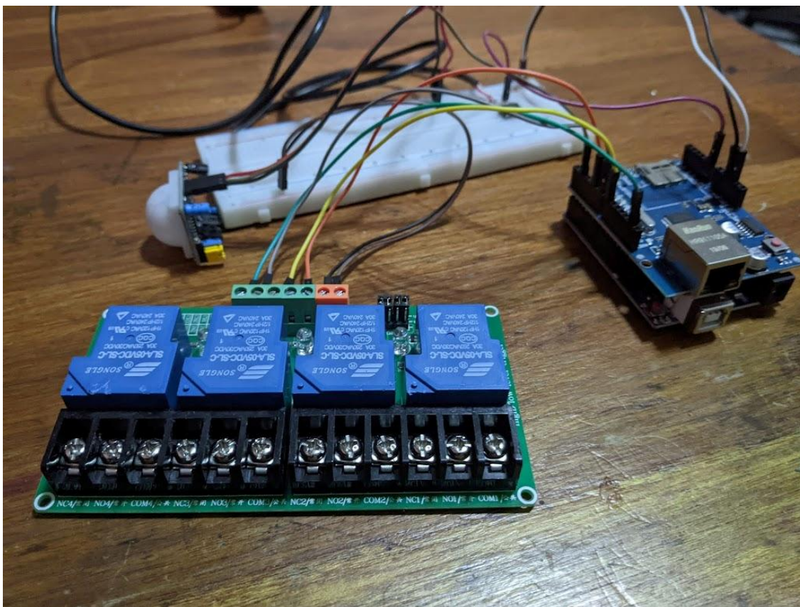
Figura 8.26 Montaje del controlador de dispositivos Stand-by en el prototipo
