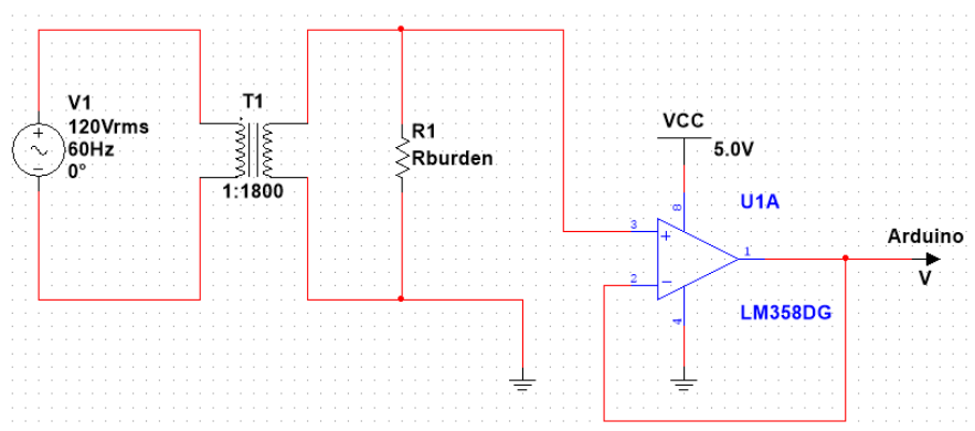
Figura 6.4 Conexión del LM358 para obtener la corriente.
