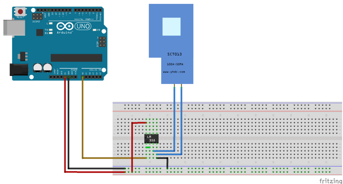
Figura 8.19 Conexión del sensor STC-013 con el Arduino
