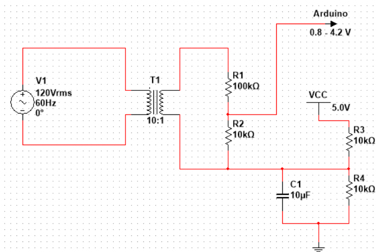
Figura 6.3 Conexión del transformador para obtener el voltaje.
