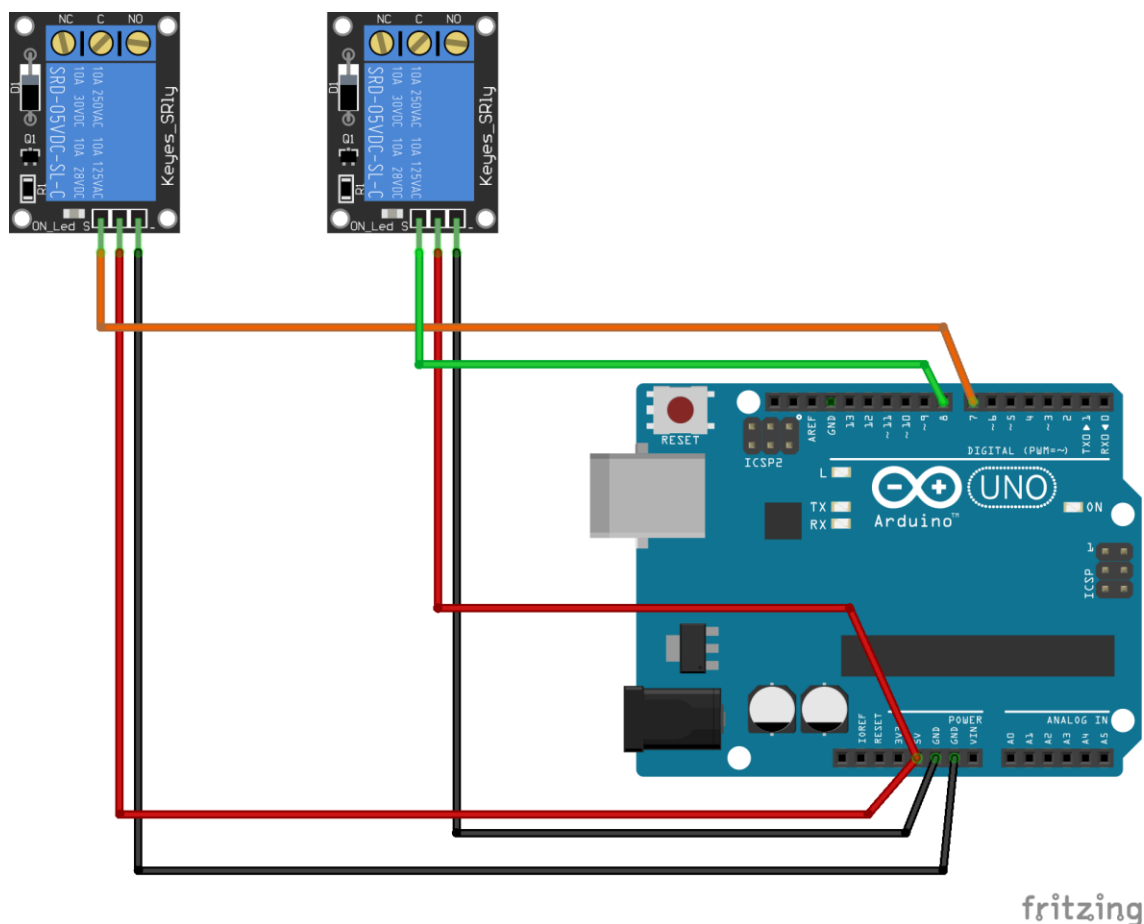
Figura 8.25 Conexión del módulo relé con Arduino
