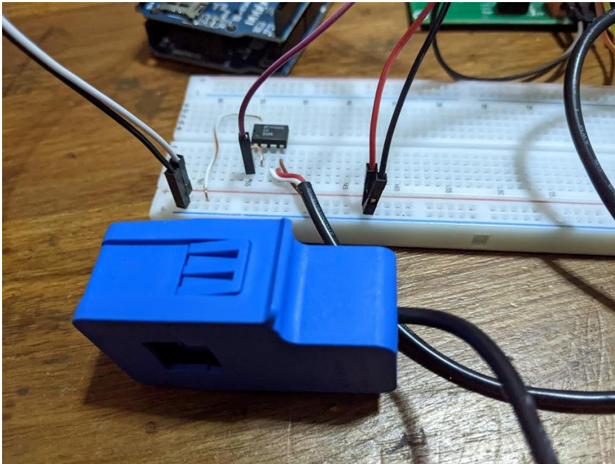
Sensor de corriente SCT-013 30
