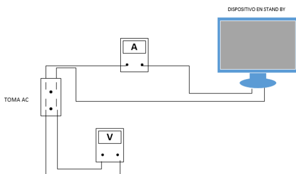
Figura 6.8 Diagrama para medición de voltaje y corriente
