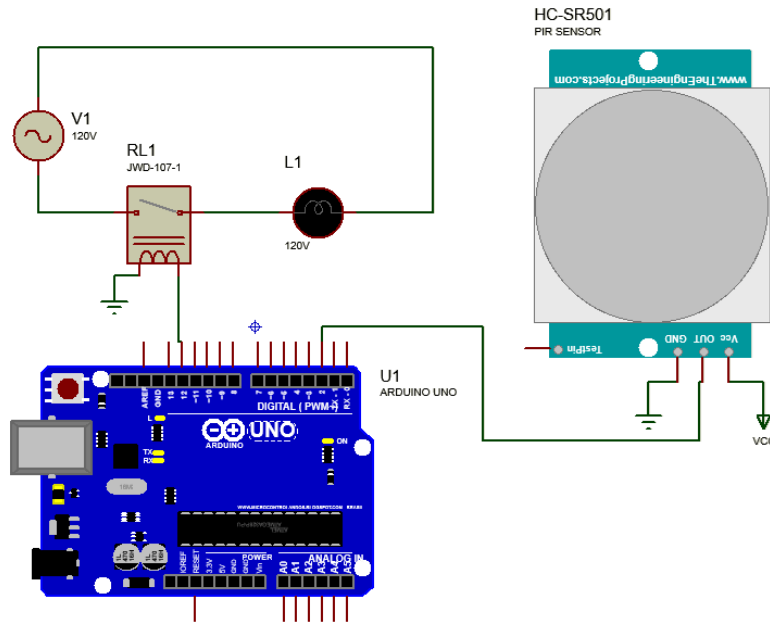
Figura 6.5 Conexión del circuito controlador de luces
