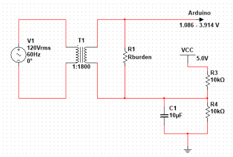
Figura 6.2 Conexión del sensor de corriente SCT-013 30
