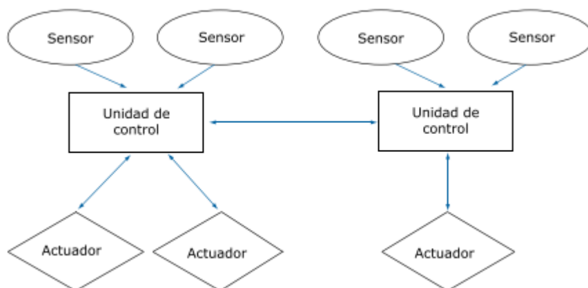
Figura 4.5 Sistema de control descentralizado
